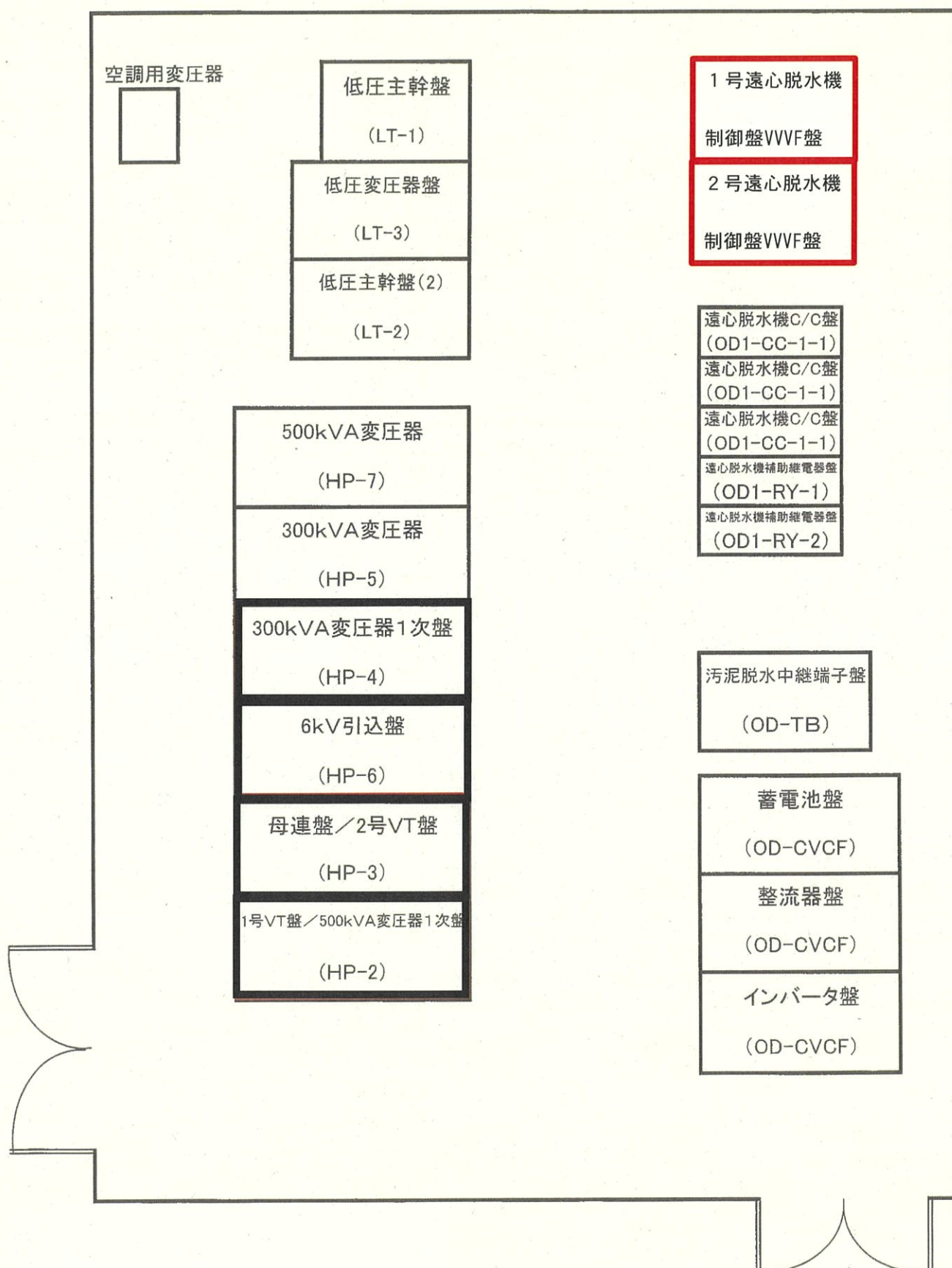
図番一 3 污泥处理棟新電気室 配置図
