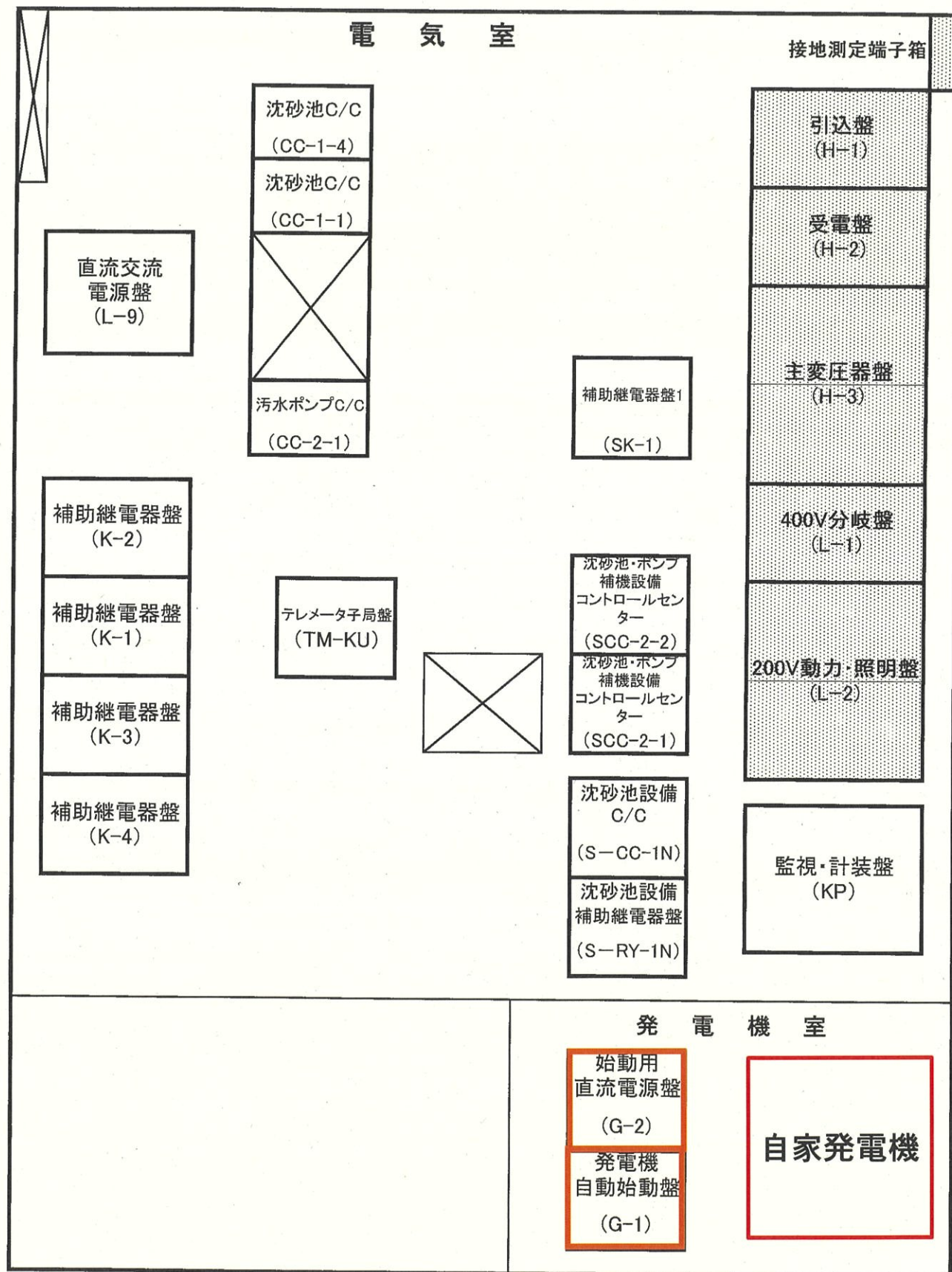
図番ー 8 栗橋中継ポンプ場 配置図
