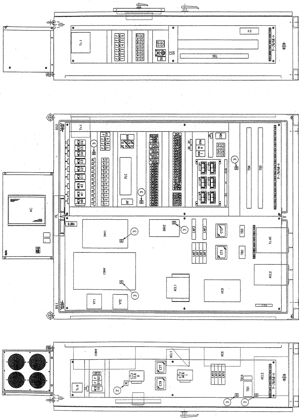
右側面内部配线图
