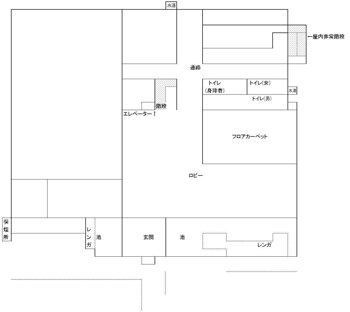
図面名 管理本館1階平面図 図番 1
