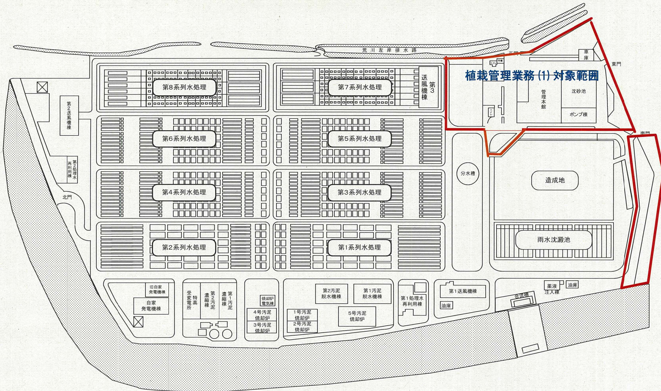
図面名 荒川水循環センター平面図 図番1
