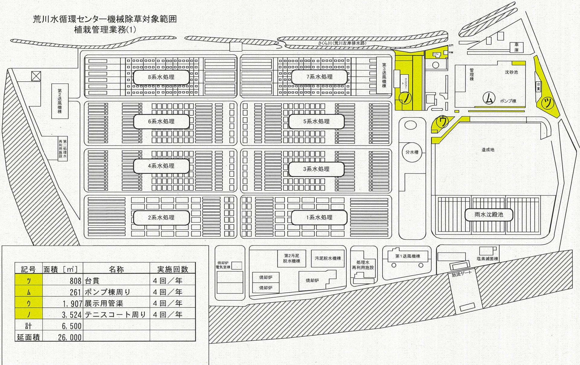
図面名 植栽管理図(機械除草) 図番3
