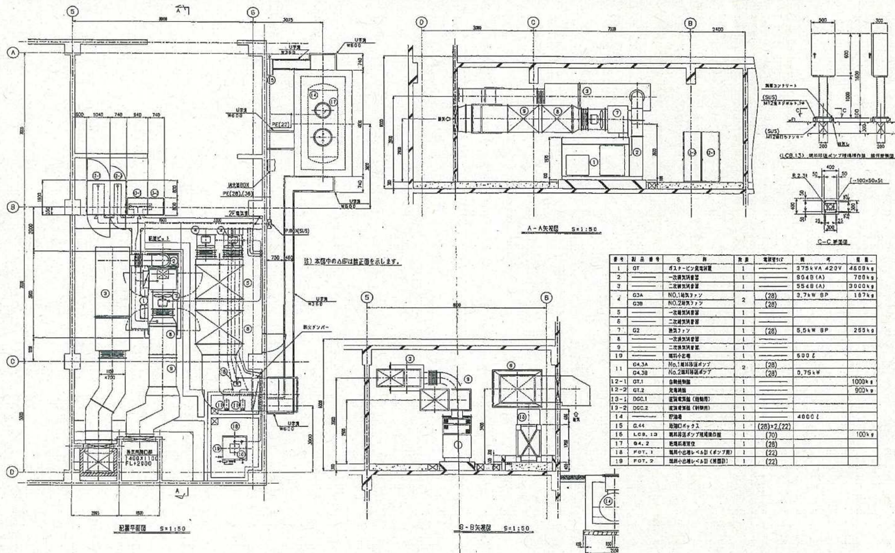
図面名 ガスタービン発電装置室 機器配置図 図番3
