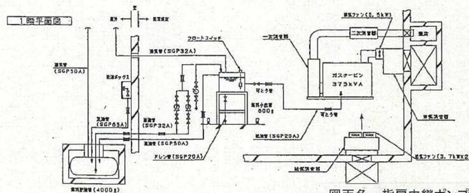
図面名 指扇中継ポンプ場 1階平面図 図番2
